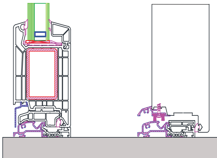
SOLUZIONE STANDARD ADOTTATA
