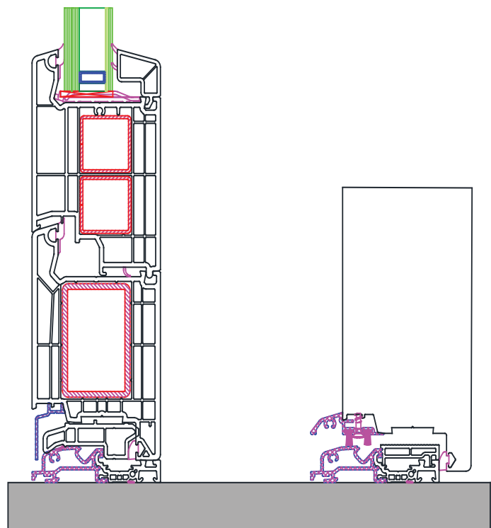
SOLUZIONE CON INSERIMENTO DI UNA ZOCCOLATURA INFERIORE
