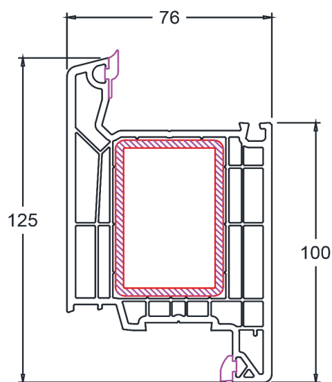
Art. 105.400 - battente per portoncini Colori: vedere tabella
