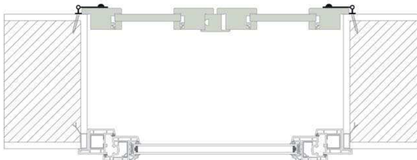
Schema di applicazione dello Scura in battuta sullo spigolo esterno.
