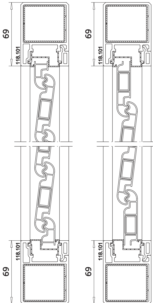
Sezione B-B
