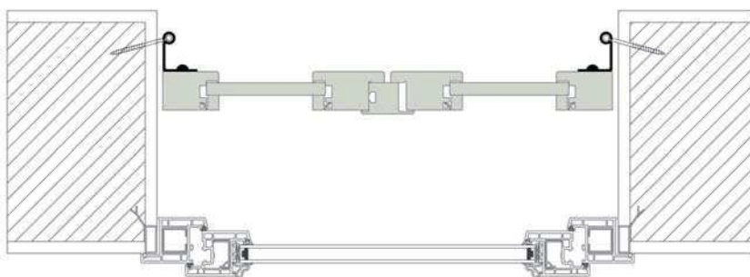
Schema di applicazione dello Scura all'interno della spalletta.
