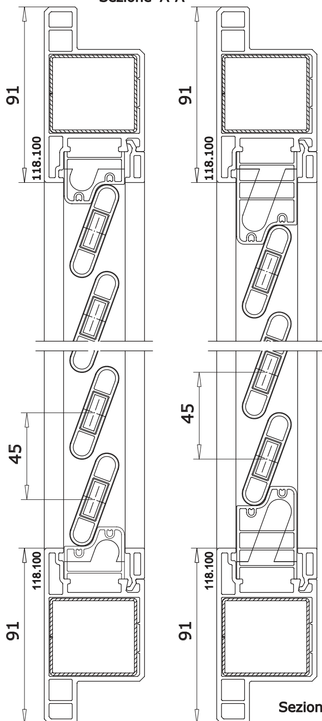
Sezione A-A
