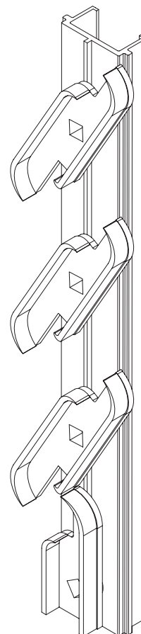
Meccanismo per orientabile VEKA (comando a pomolo (solo colore NERO))
