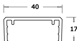
Art. 118.064 Profilo a "C" di copertura
