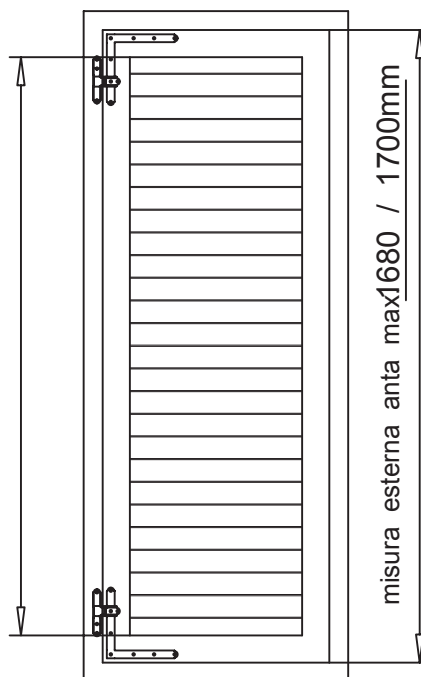
Meccanismo per orientabile VEKA (comando a pomolo (solo colore NERO))
