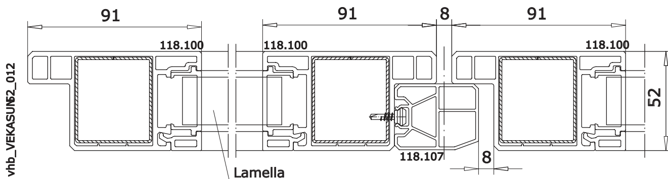
Sezione B-B
