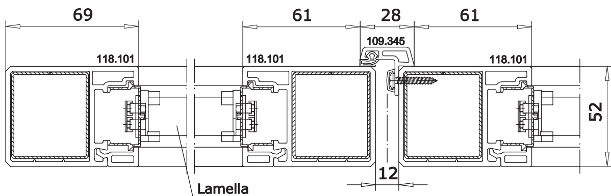
Sezione B-B
